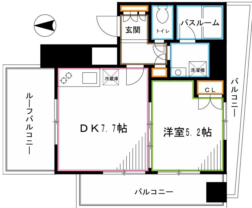
【間取り図】
