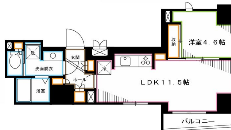
【間取り図】
