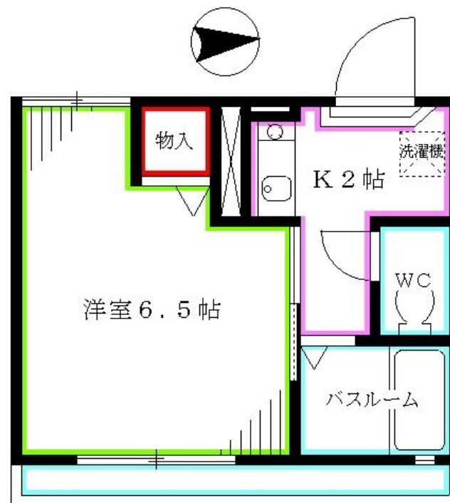
【間取り図】
