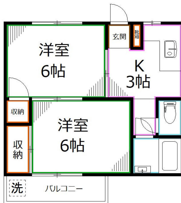
【間取り図】
