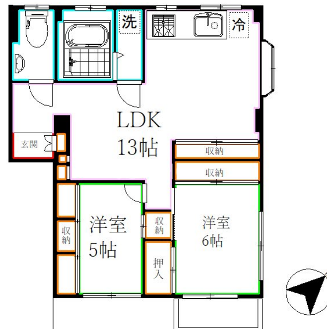
【間取り図】
