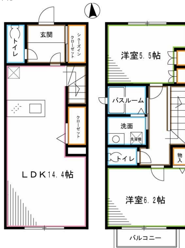
【間取り図】
