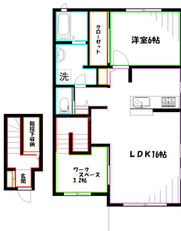
【間取り図】
