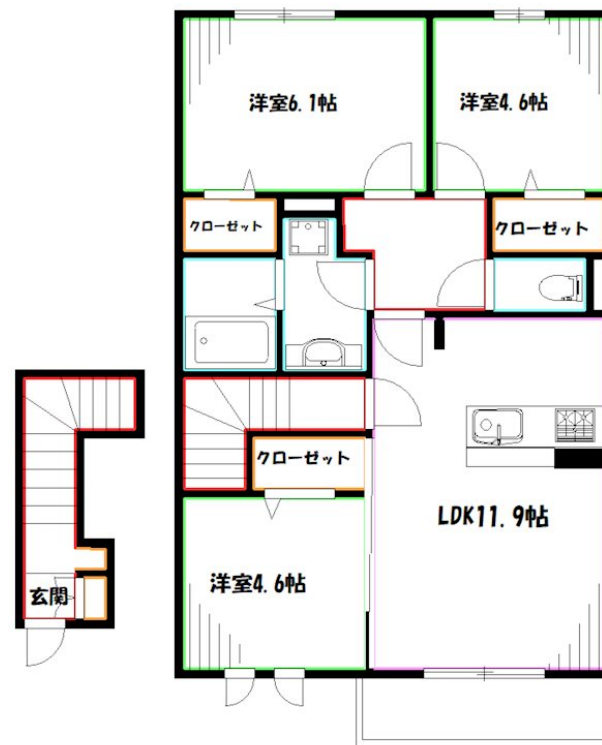
【間取り図】
